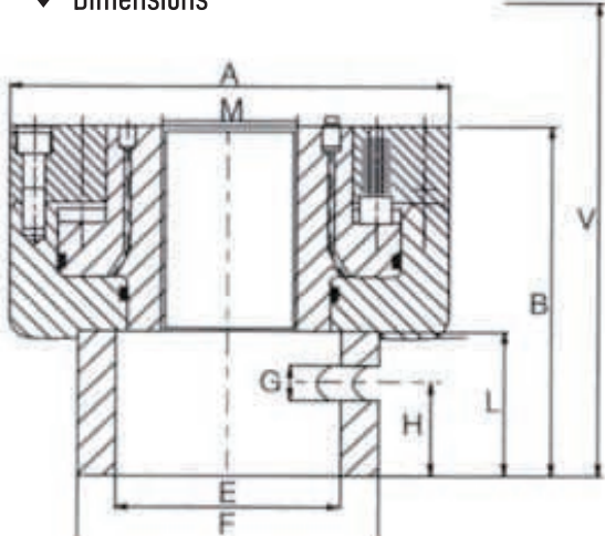
▼ Dimensions
